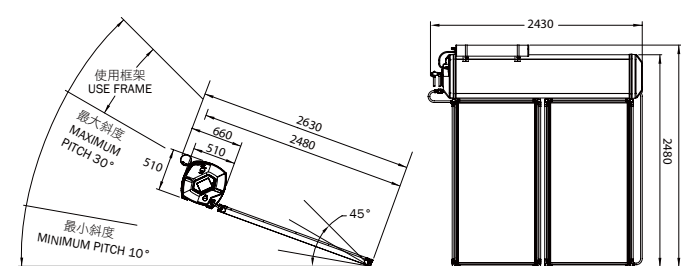
安裝尺寸 Installation Dimensions (mm)
