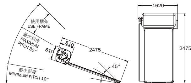
安裝尺寸 Installation Dimensions (mm)
